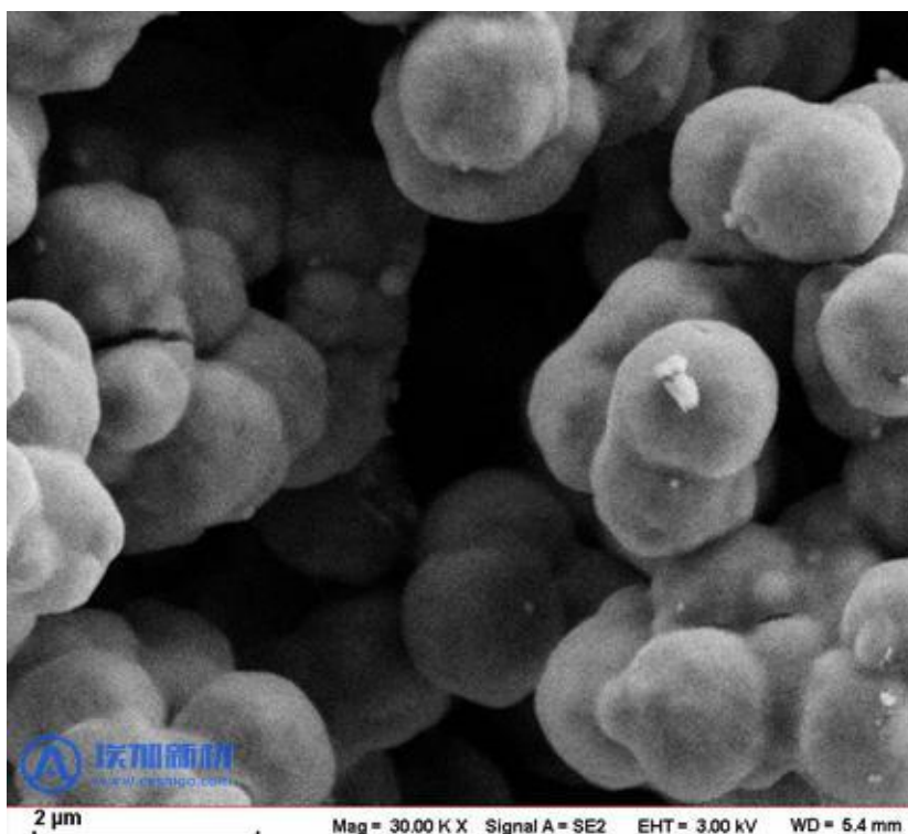
图 2 二氧化钛磁珠（厚壳层）的扫描电镜图
