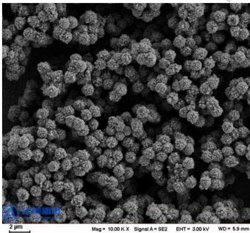
图 1 二氧化钛磁珠（薄壳层）的扫描电镜图
