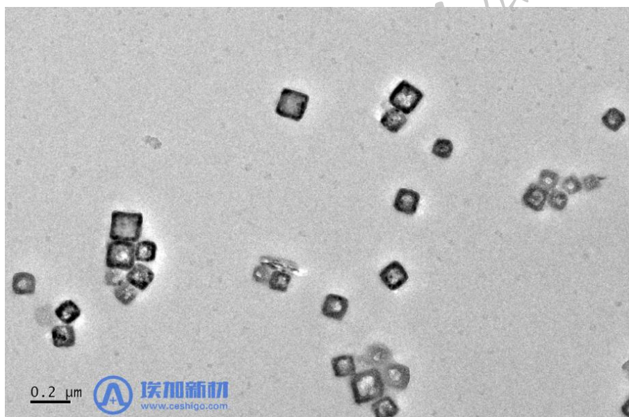
图 1 中空介孔普鲁士蓝纳米颗粒的透射电镜图
