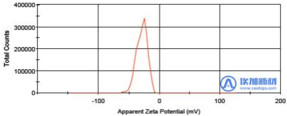
图 2 羧基磁珠 Zeta 电位
