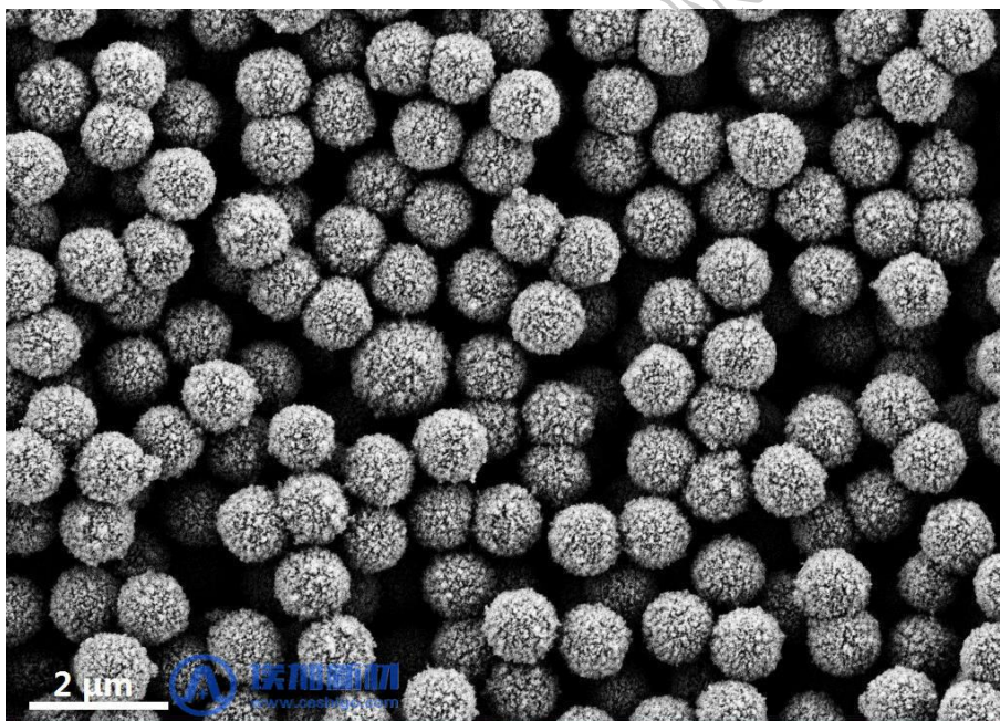
图 1 羧基磁珠的扫描电镜图
