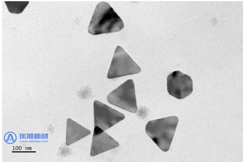
图 2 水溶性金纳米三角片的透射电镜图
