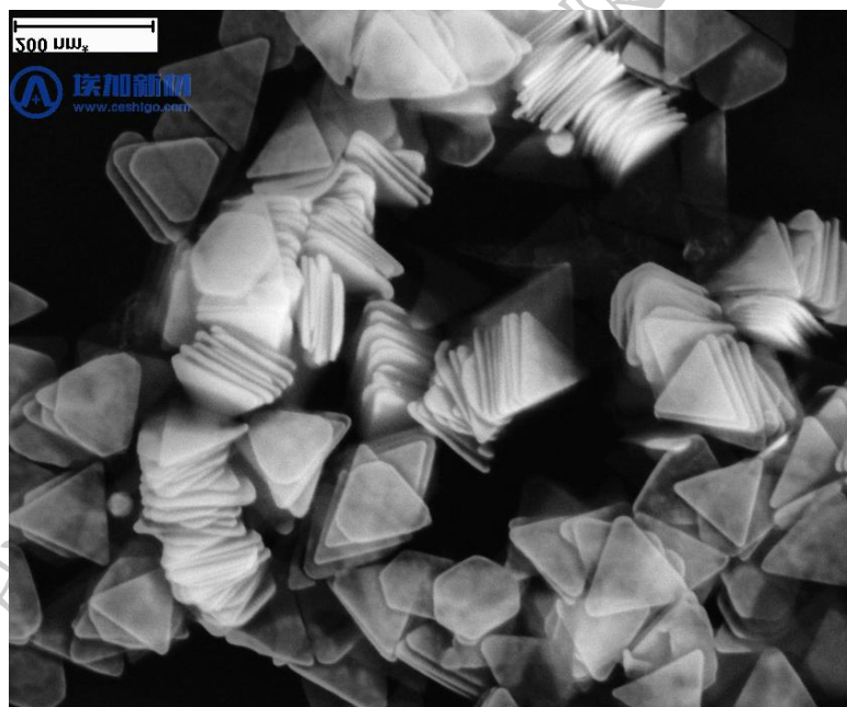
图 1 水溶性金纳米三角片的扫描电镜图
