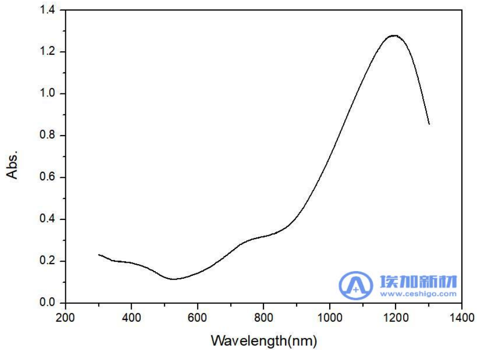
图 3 水溶性金纳米三角片的紫外-可见光吸收谱图
