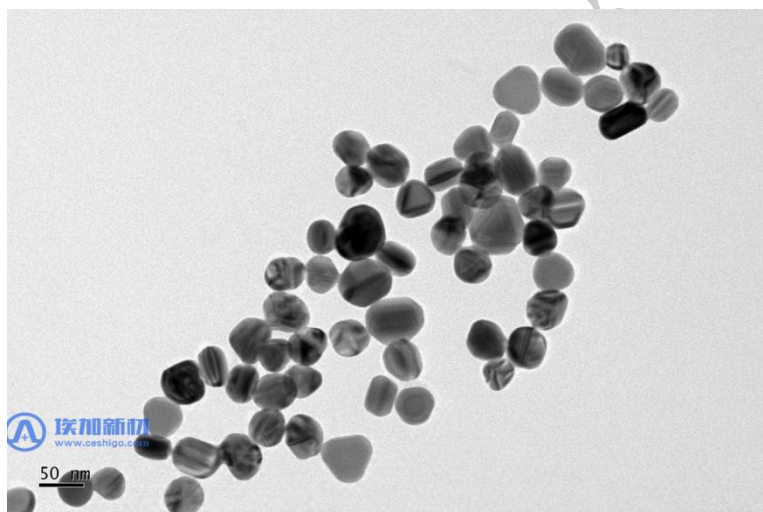
图 1 水溶性银纳米颗粒 (50nm) 的透射电镜图
