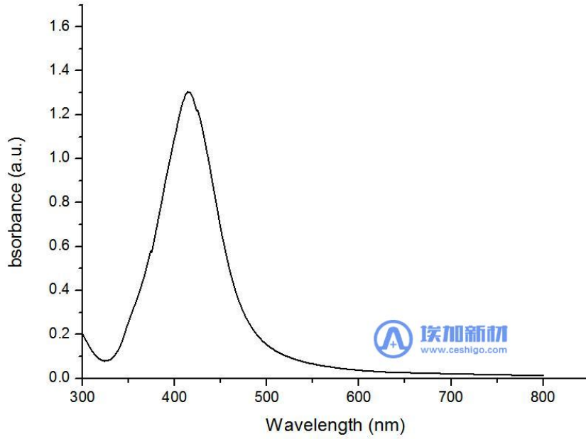
图 2 水溶性银纳米颗粒 (40nm) 的紫外-可见光吸收谱图
