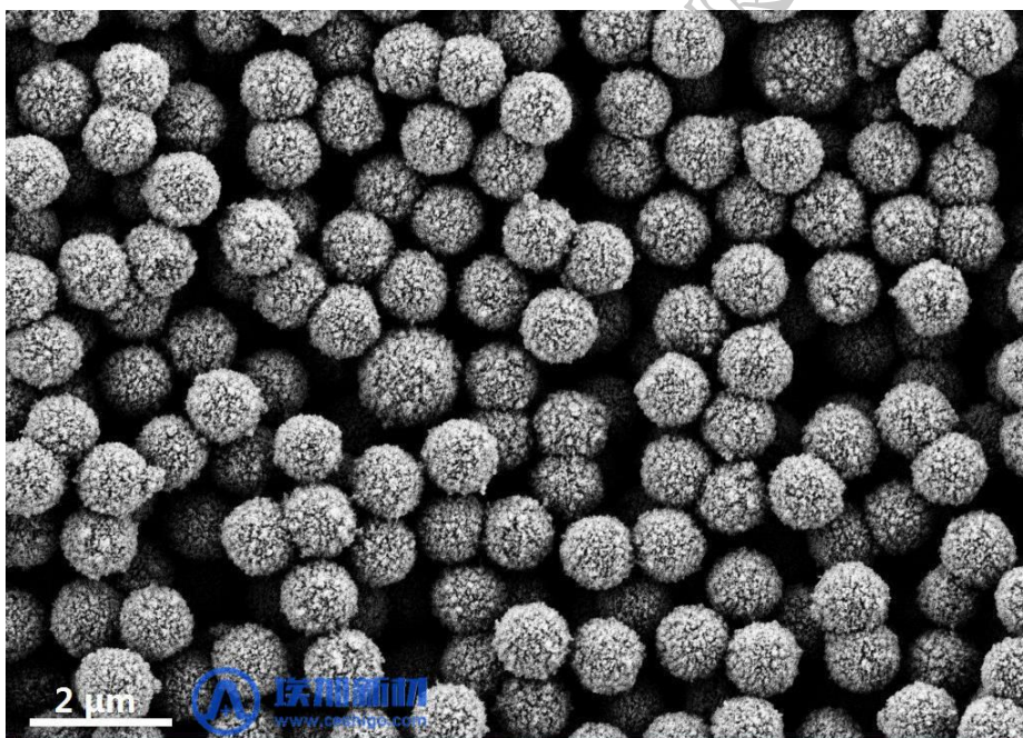
图 1 氨基磁珠的扫描电镜图
