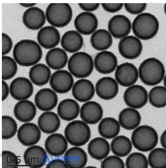
图 4 中空介孔二氧化硅（球状）400nm 的透射电镜图
