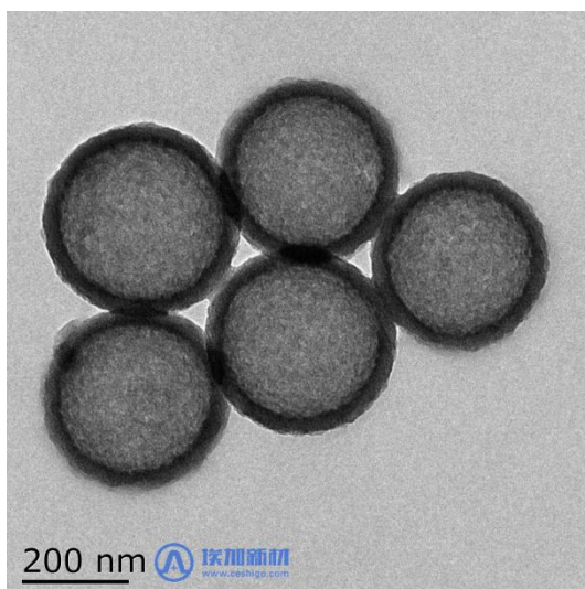
图 3 中空介孔二氧化硅（球状）300nm 的透射电镜图
