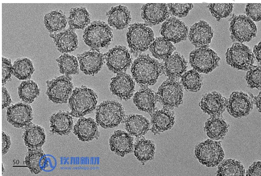
图 1 中空介孔二氧化硅溶液（球状）70±10nm 的透射电镜图
