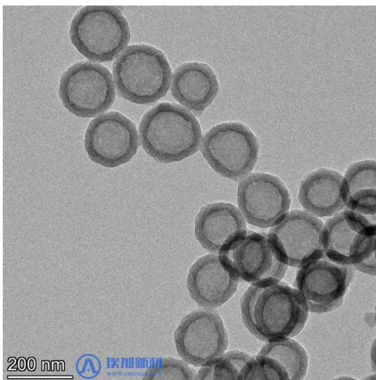
图 2 中空介孔二氧化硅溶液（球状） 160\pm 10\text{nm} 的透射电镜图
