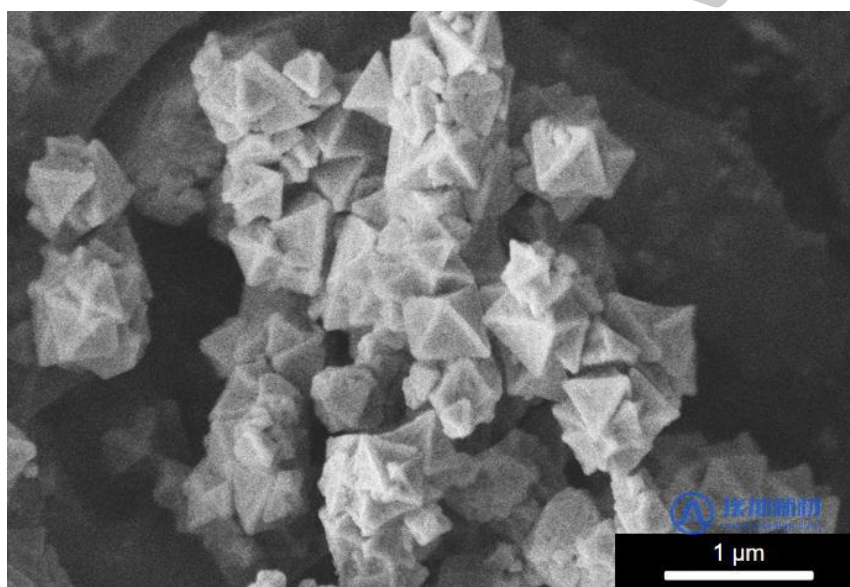
图 1 MOF-808 的扫描电镜图
