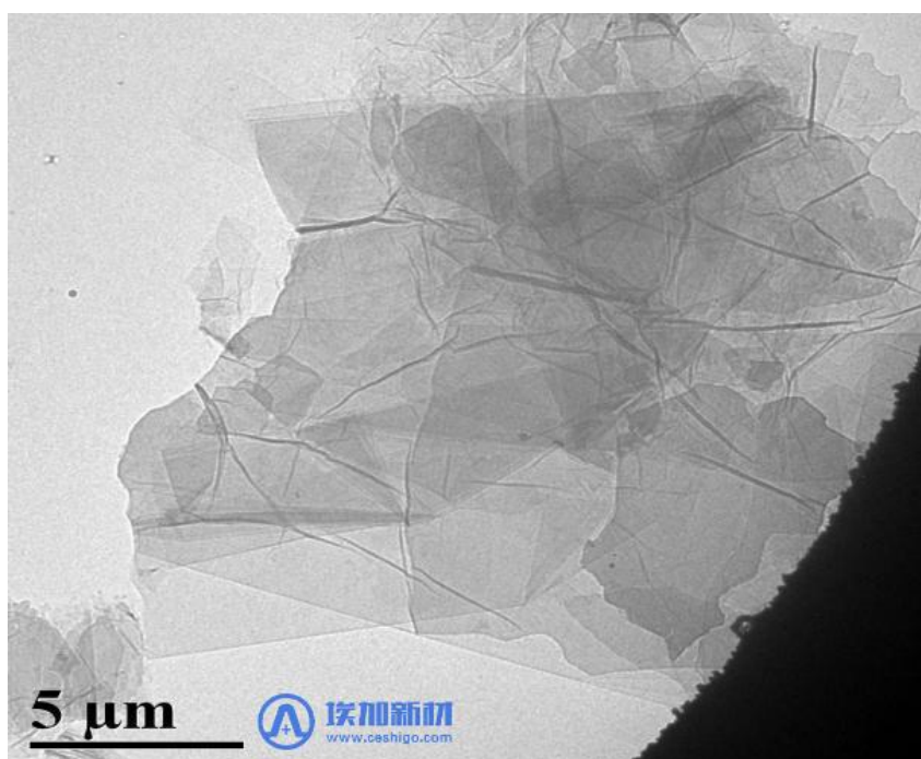
图 1 大片径氧化石墨烯的透射电镜图
