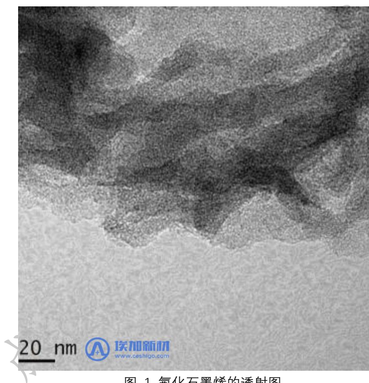
图 1 氟化石墨烯的透射图
