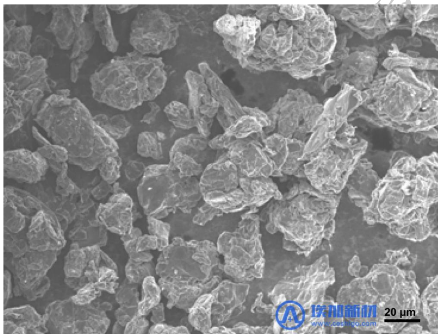
图 1 氧化石墨粉末的扫描电镜图
