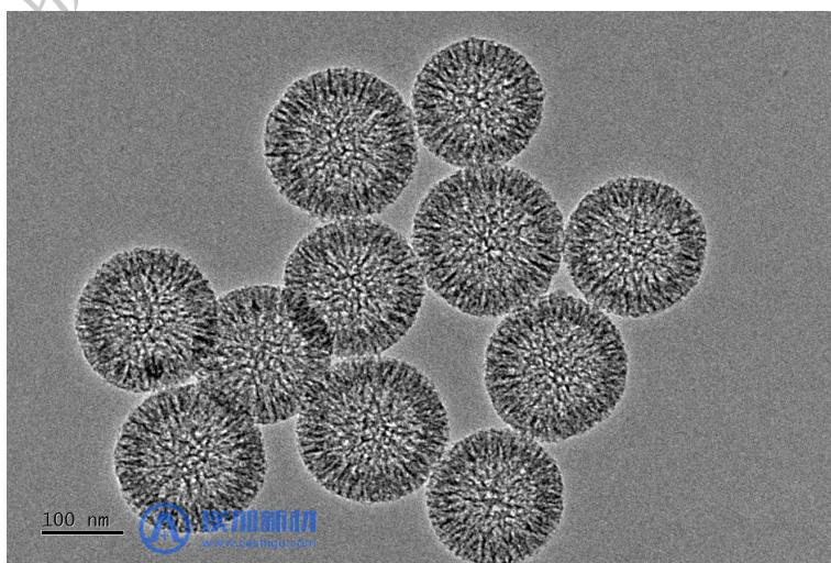
图 2 中空碳球（硬模板法）的透射电镜图
