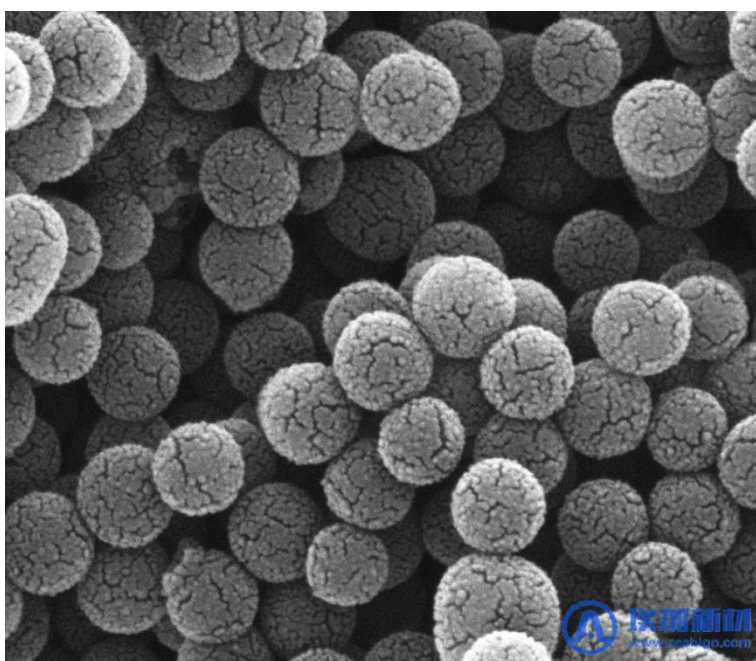
图 1 中空碳球（硬模板法）的扫描电镜图
