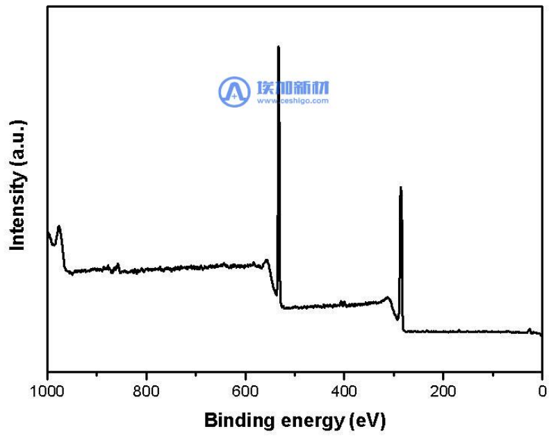
图 3 羧基化氧化石墨烯粉末的 XPS 图谱
