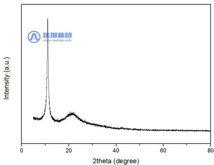
图 1 羧基化氧化石墨烯粉末的 XRD 图谱
