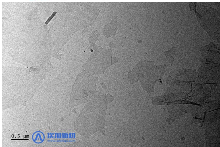
图 5 羧基化氧化石墨烯分散液 片径<500nm 的透射图
