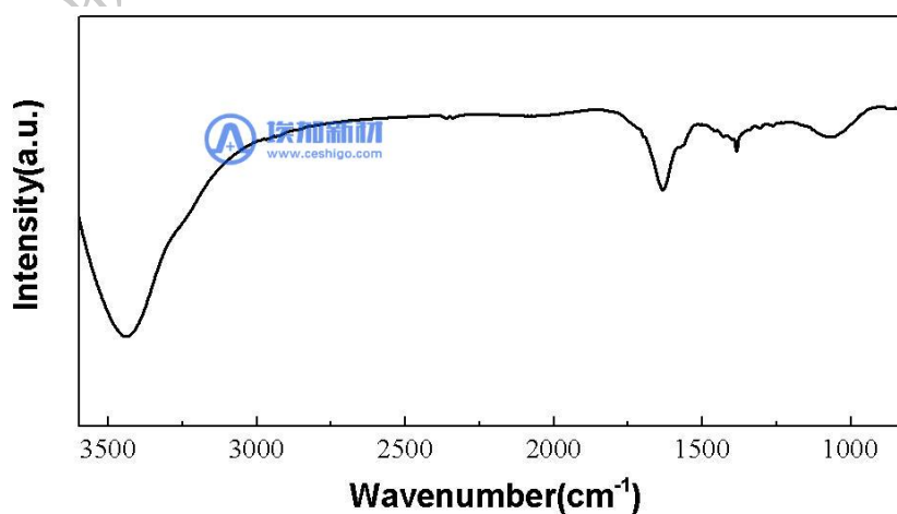
图 2 羧基化氧化石墨烯粉末的红外图谱
