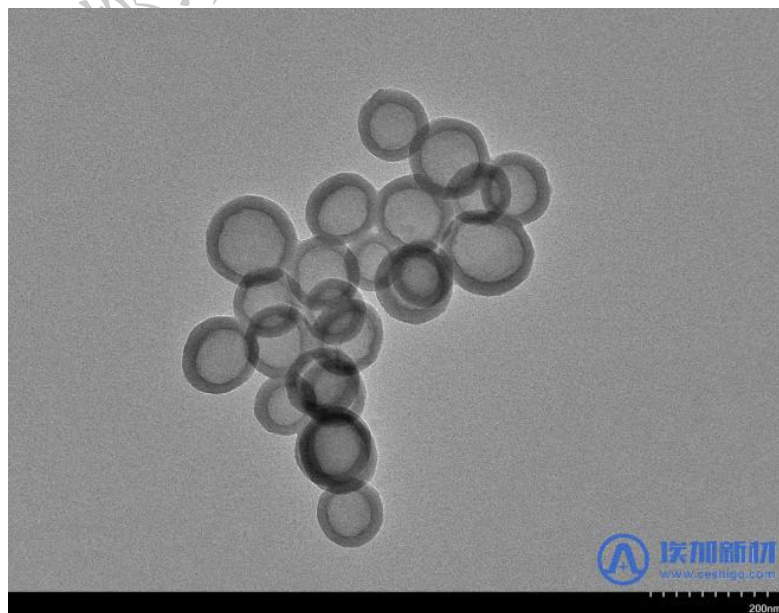
图 2 中空碳球（软模板法）90-150nm 的透射电镜图
