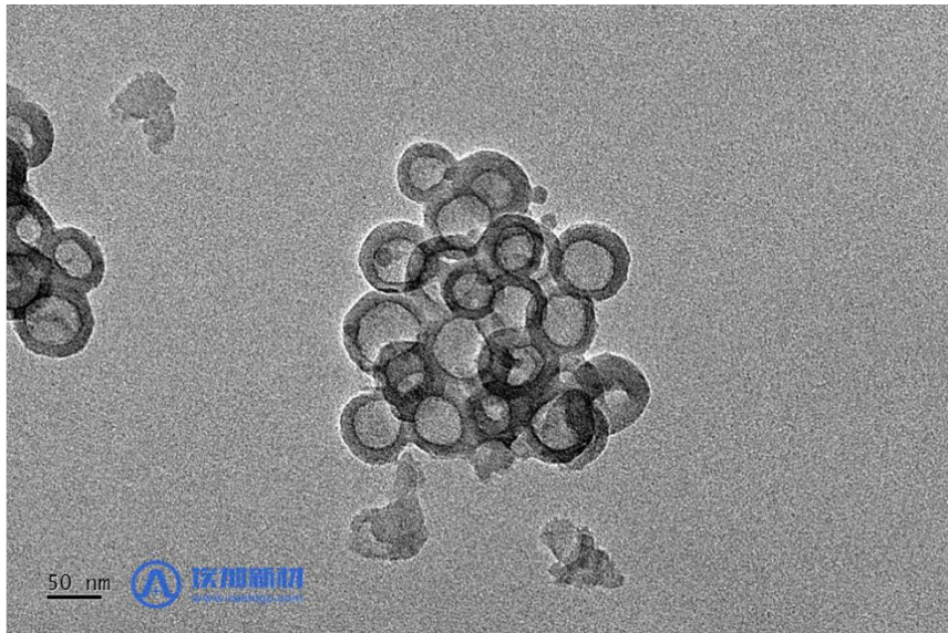
图 1 中空碳球（软模板法）50-80nm 的透射电镜图
