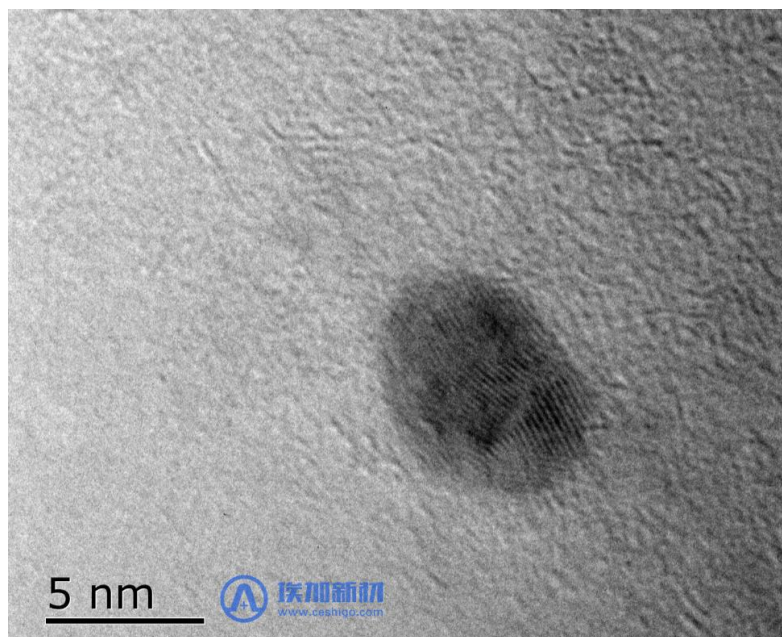
图 2 黑磷量子点分散液的透射电镜图
