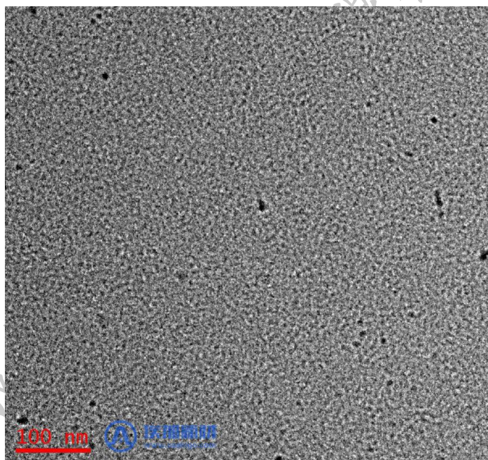
图 1 黑磷量子点分散液的透射电镜图
