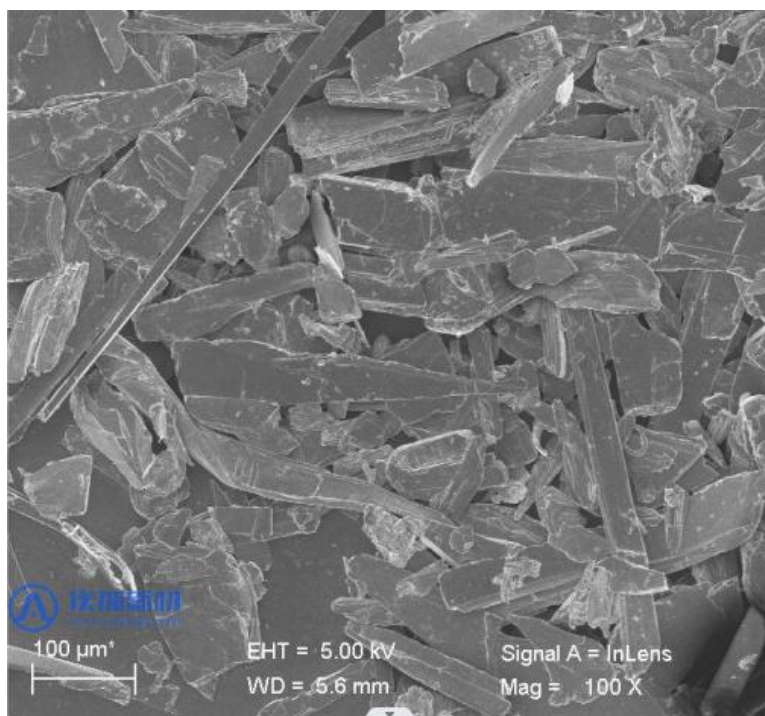
图 1 黑磷晶体粉末的扫描电镜图
