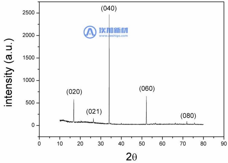
图 2 黑磷晶体粉末的 XRD 图
