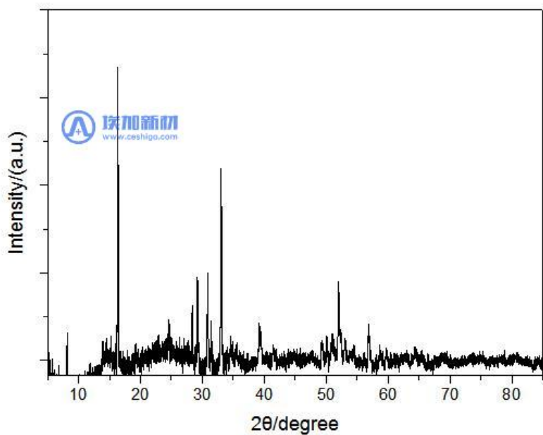
图2 紫磷晶体的 XRD 图谱
