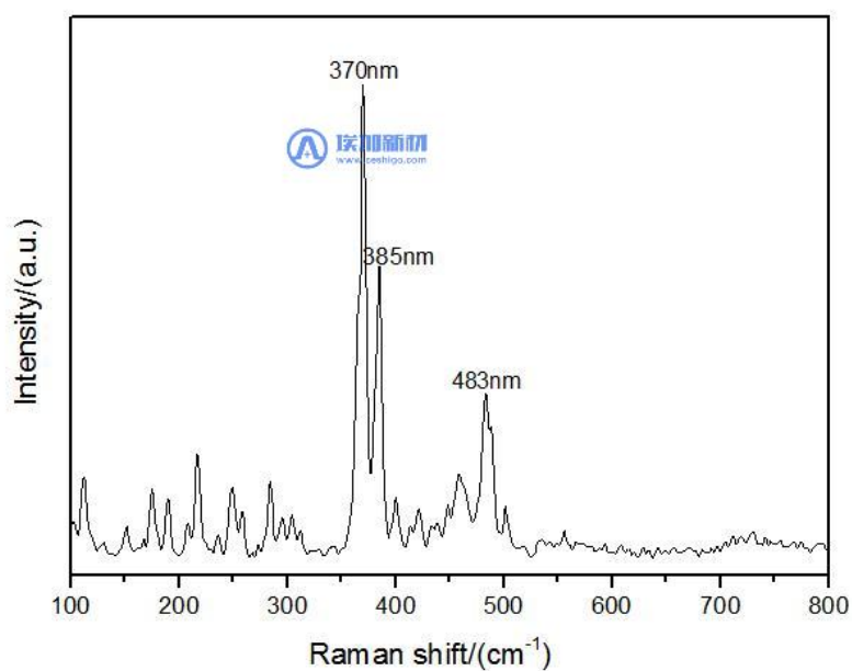
图3 紫磷晶体的拉曼图谱
