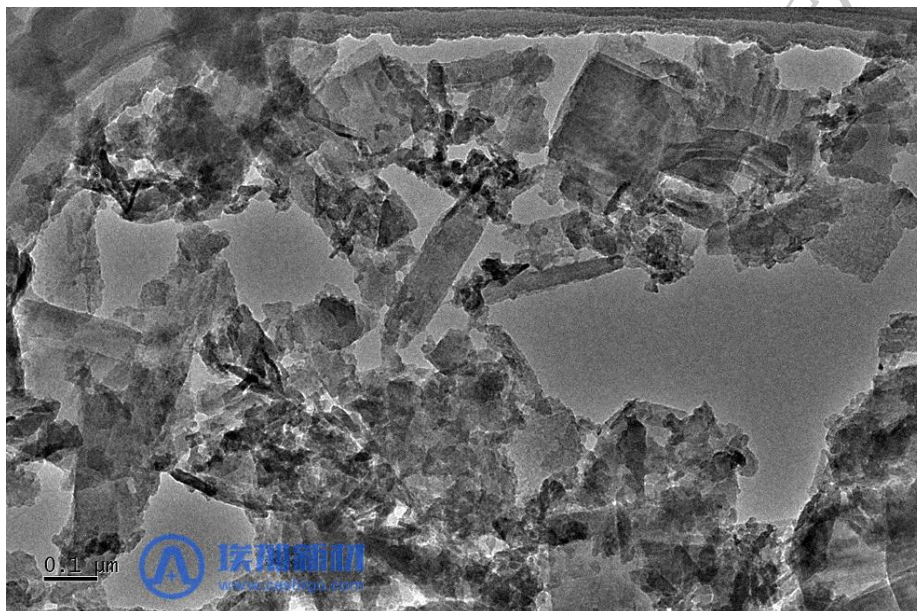
图 1 紫磷纳米片分散液的透射电镜图
