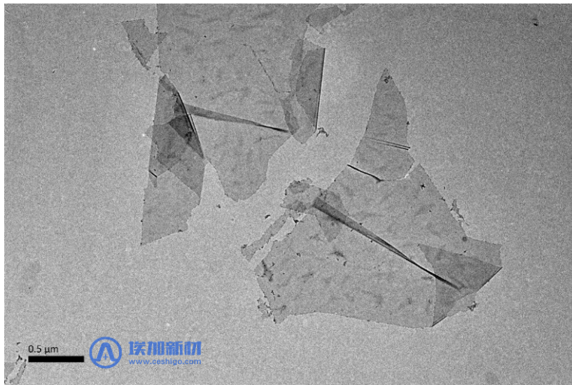
图 1 Ti3C2Tx 少(单)层分散液的 TEM 图
